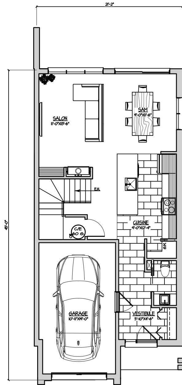
REZ-DE-CHAUSSÉE LOGEMENT C SUPERFICIE BATIMENT: 901 P.C.A.
