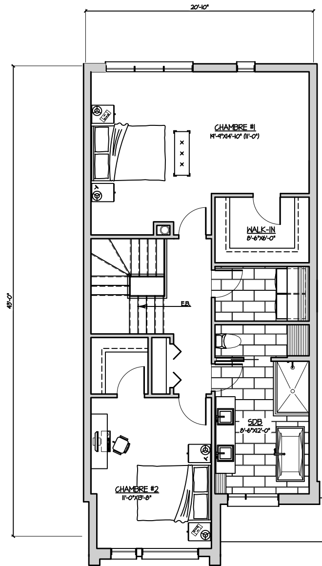
ÉTAGE OPT 2CH. LOGEMENT C SUPERFICIE BATIMENT: 688 P.C.A.
