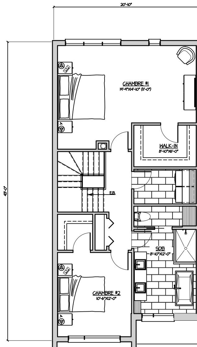
ÉTAGE OPT 2CH. LOGEMENT A
