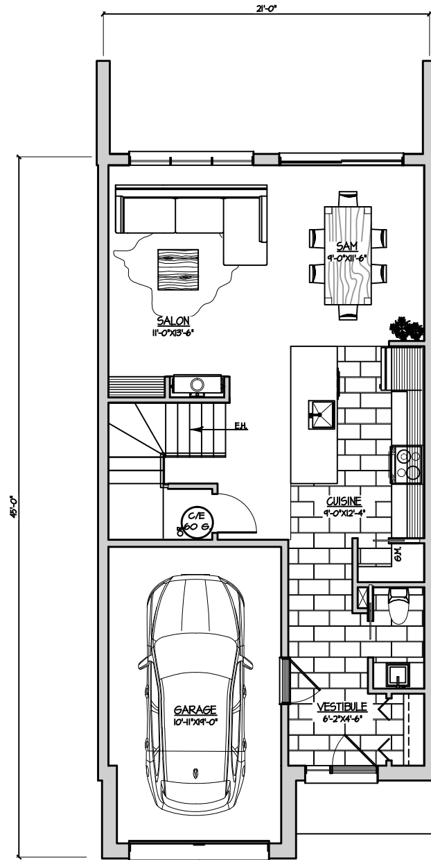
REZ-DE-CHAUSSÉE LOGEMENT B
